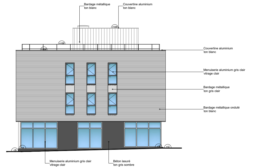
FACADE SUD OUEST
