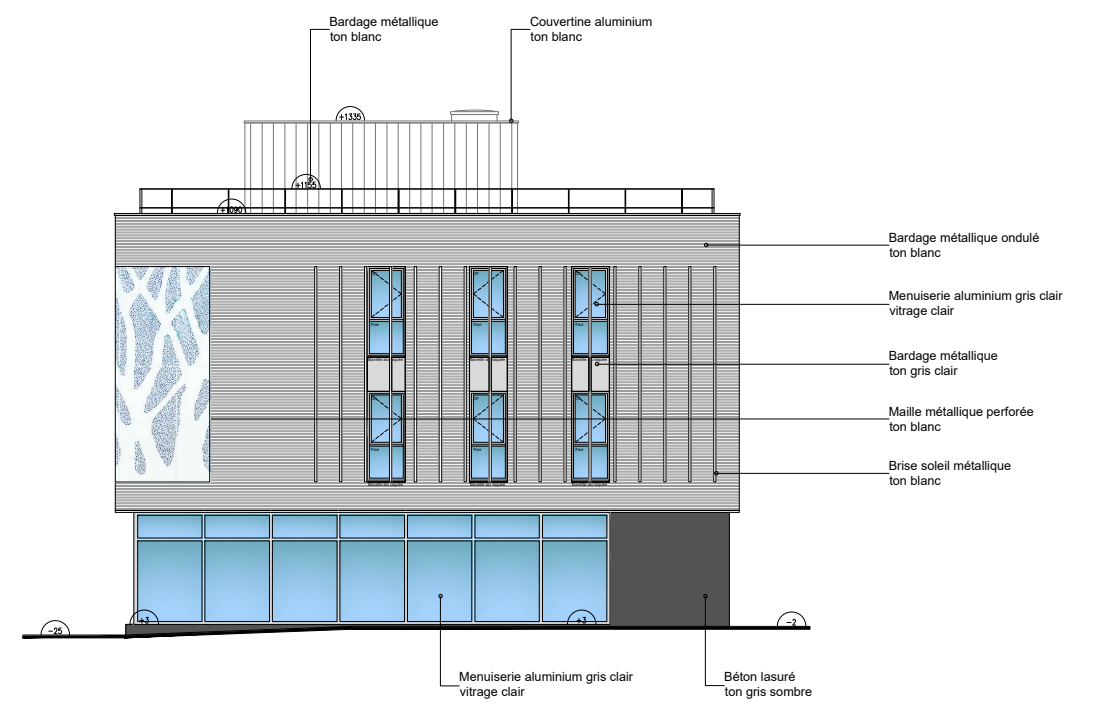
FACADE NORD EST
